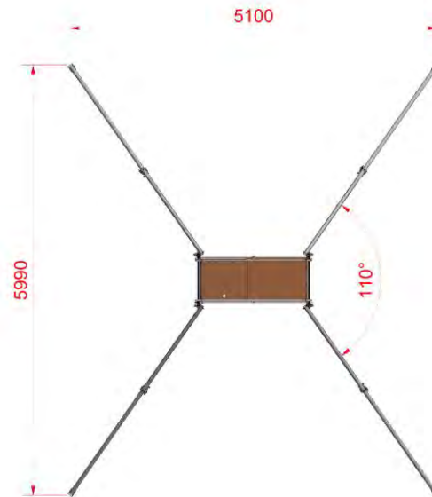
Draufsicht
