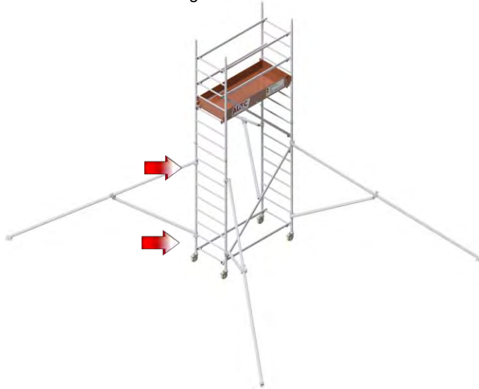
Seitenansicht
